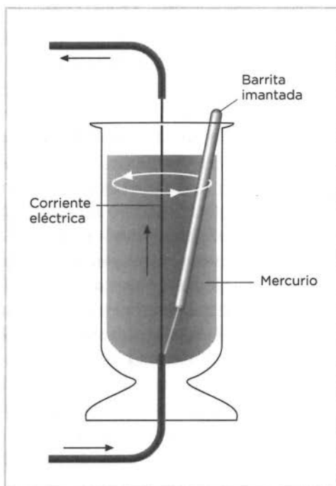
El primer motor eléctrico de Faraday, construido en 1821.
